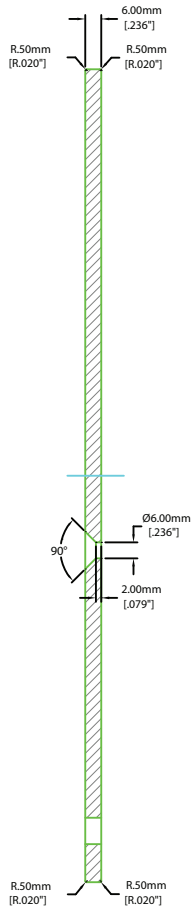
SECTION A-A
